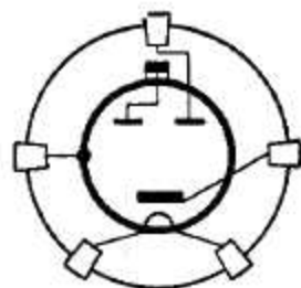
Sockelschaltung
